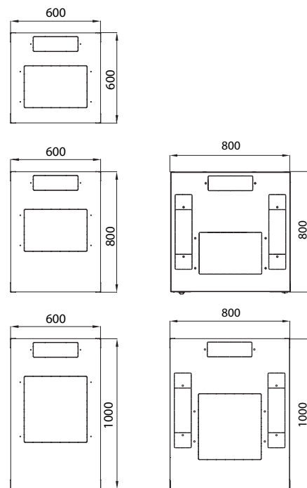
HORNÍ POHLED
